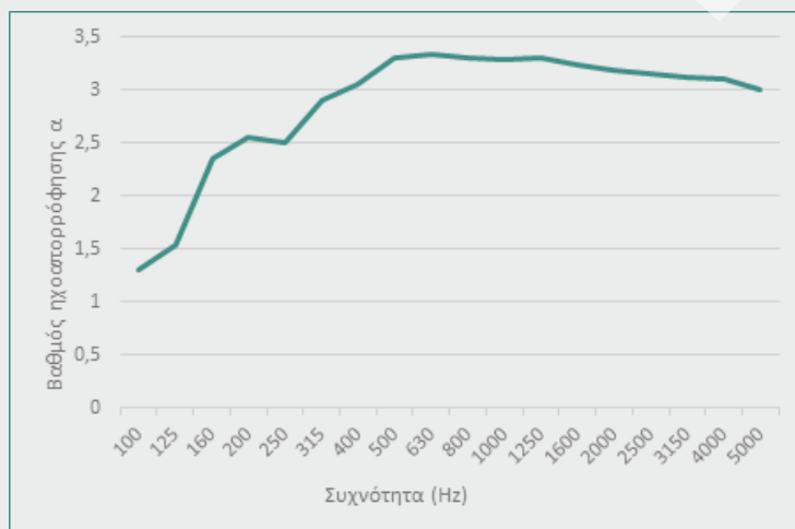
Δείκτης ηχοαπορρόφησης βάσει UNI EN ISO 354. Διαστάσεις δείγματος: 40,0 x 40,0 x 180,0cm
